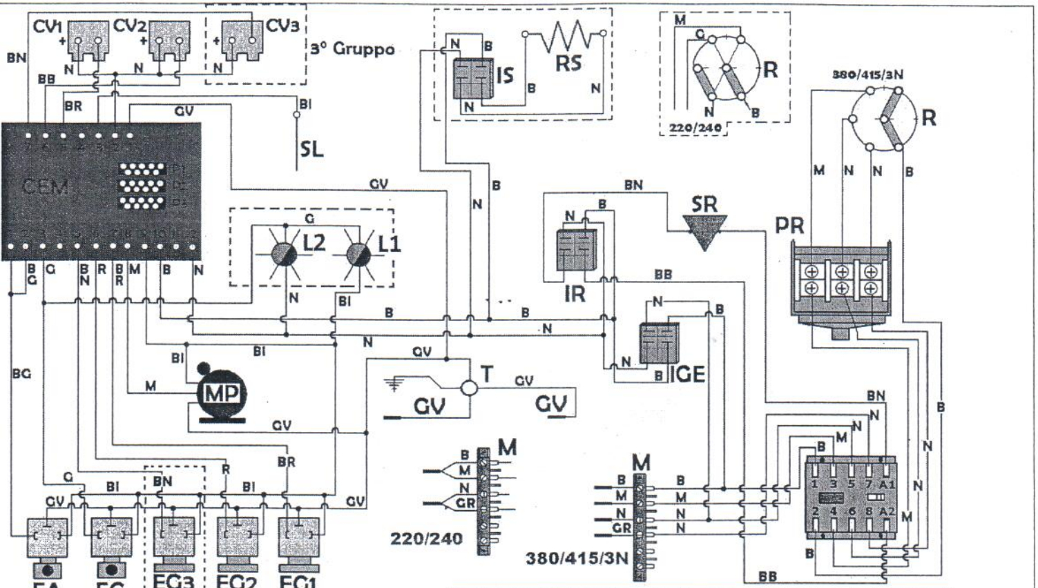
Schema elettrico ES 100/2 - 3 cavo 5 capi
